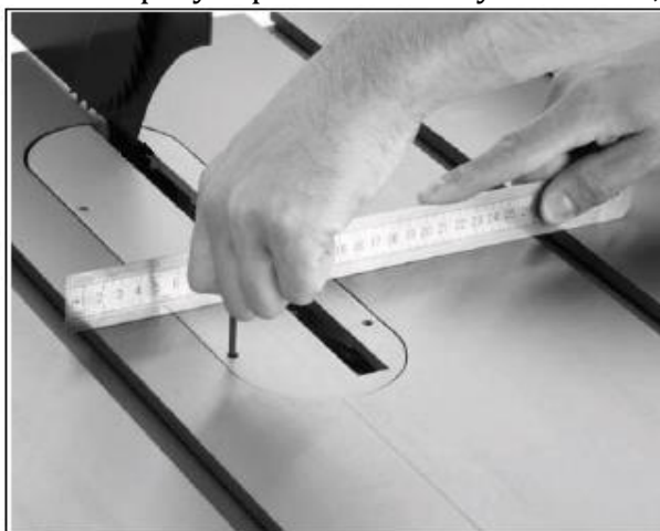
Рис. 23. Регулировка вставки стола по высоте
