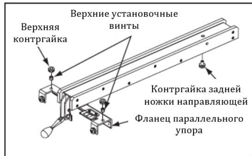
Рис. 39. Элементы параллельного упора, используемые для регулировки параллельного упора по высоте и перпендикулярности относительно стола
