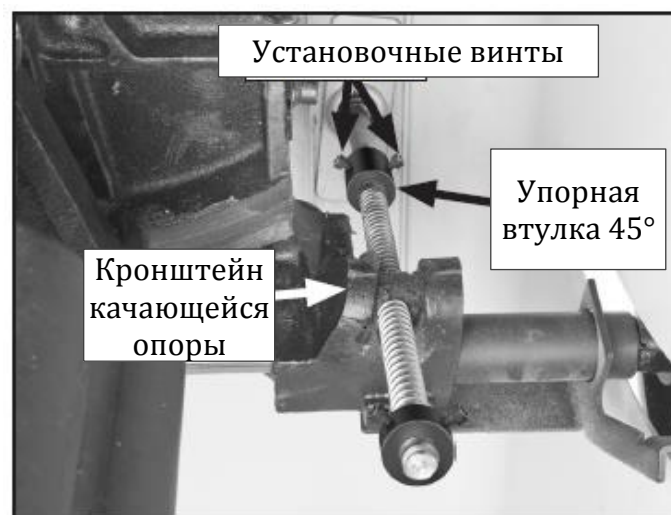
Рис. 66. Упорная втулка 45°
