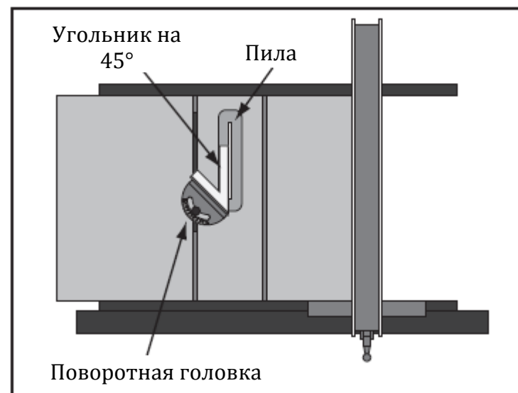
Рис. 84. Проверка положения упора на 45^\circ на поворотной головке
