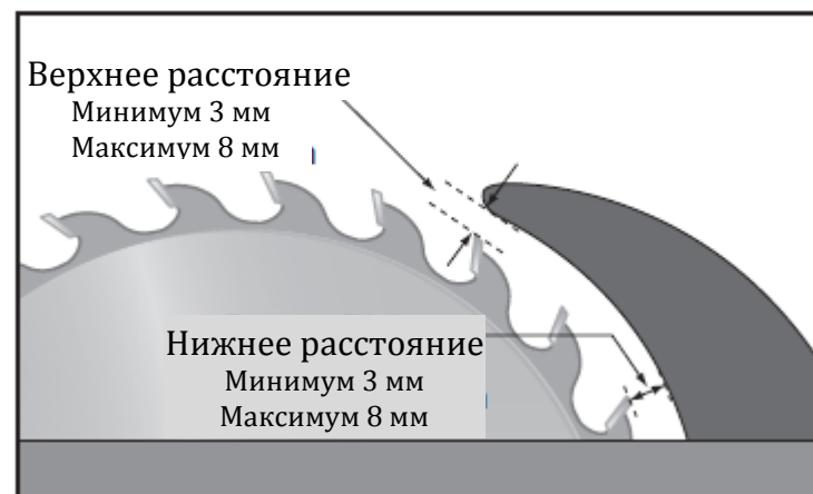
Рис. 41. Допускаемые верхнее и нижнее расстояния между расклинивающим ножом и диском пилы
