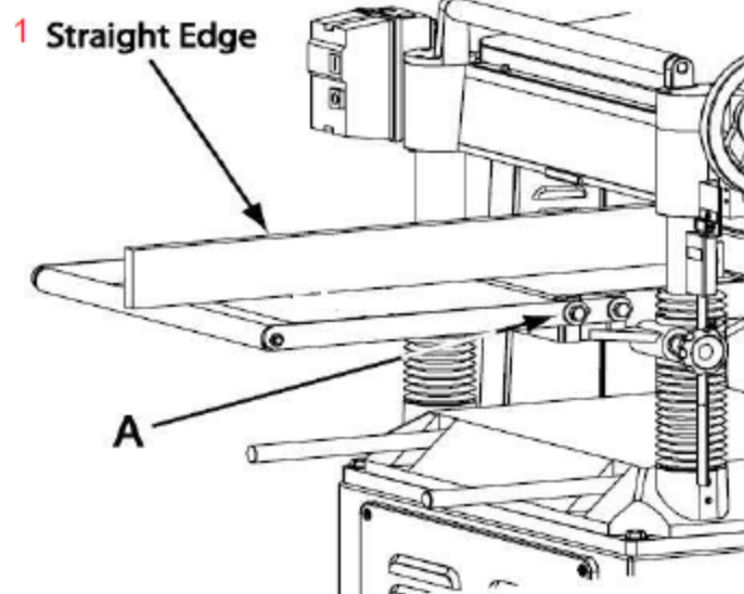
Рис. 15: 1 – поверочная линейка
