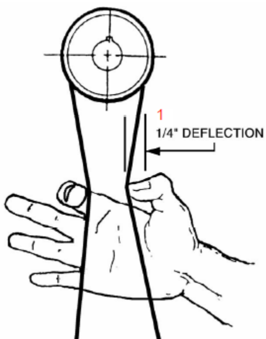
Рис. 10:1 – прогиб 6,4 мм
