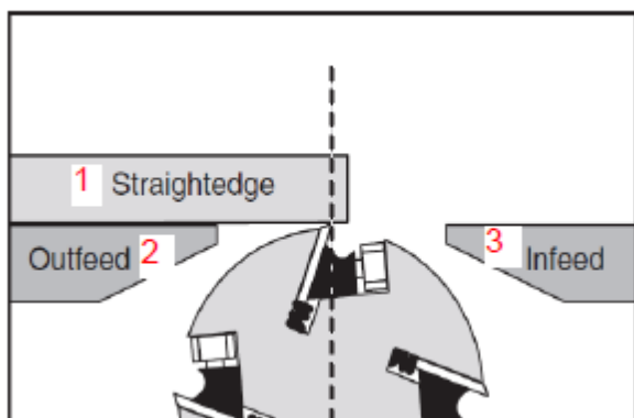
Рис. 11: 1 – поверочная линейка, 2 – отводящий стол, 3 – подающий стол
