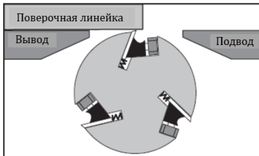
Рис. 22. Подводной стол, отрегулированный вровень с выводным столом и ножом в ВМТ
